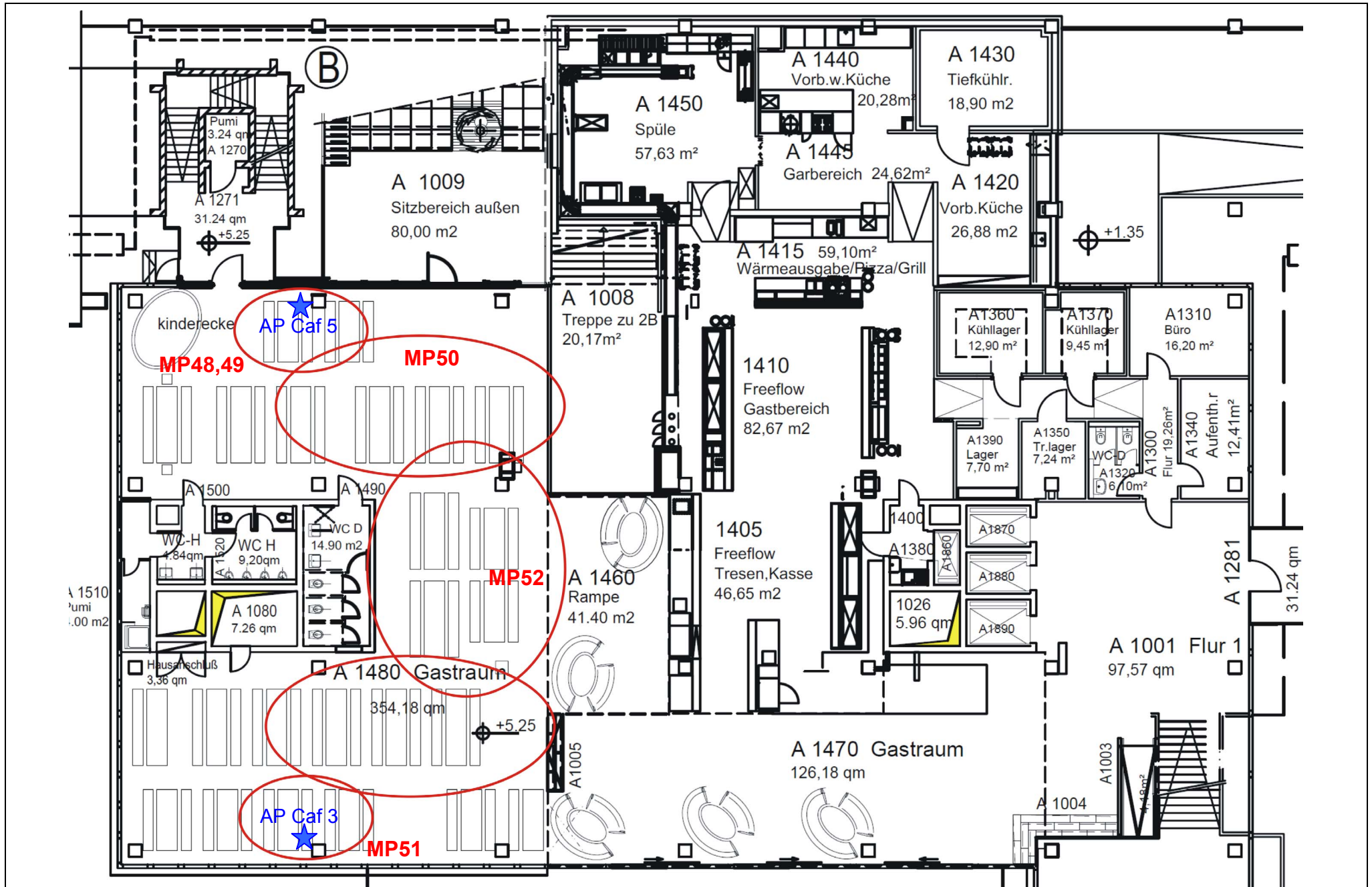
Lageplan 3: Gebäude Geisteswissenschaften 2 (GW2), Cafeteria Ebene 1, Lage der Messpunkte (MP) und Access-Points (AP)
